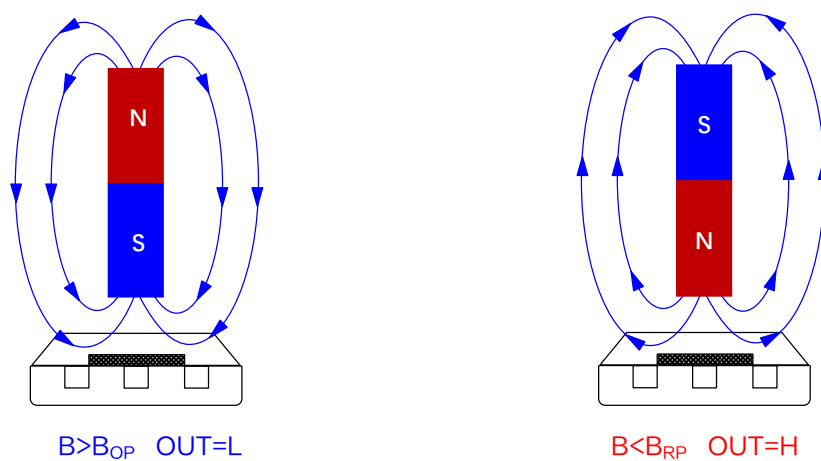
图 4.XL533 磁场方向定义图
