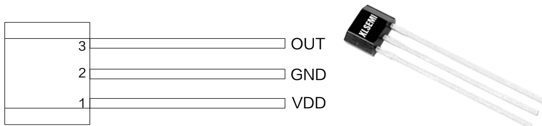
图 2.XL533 引脚配置
