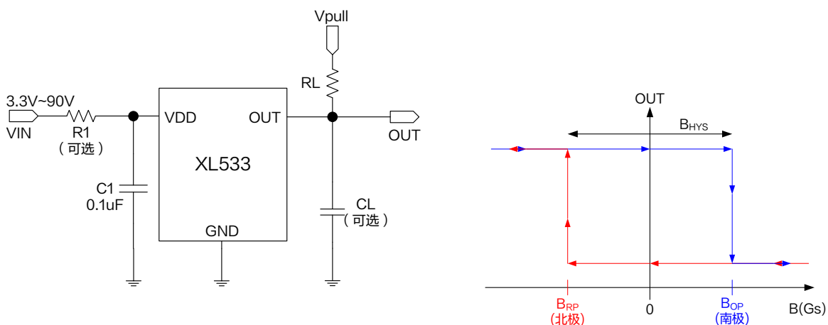
图 1.XL533 典型应用示意图和输出特性曲线
