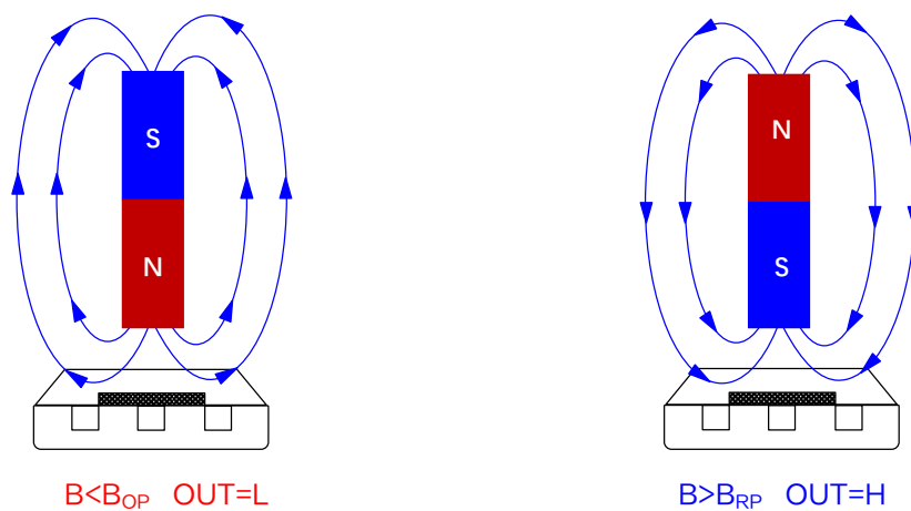
图 4.XL529 磁场方向定义图
