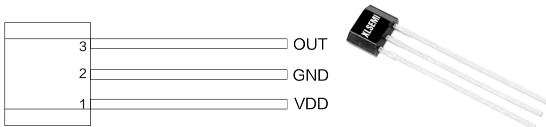
图 2.XL529 引脚配置
