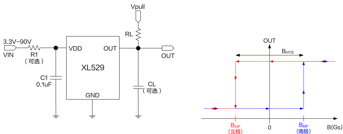
图 1.XL529 典型应用示意图和输出特性曲线
