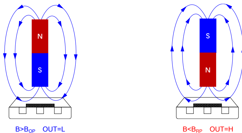
图 4. XL525 磁场方向定义图
