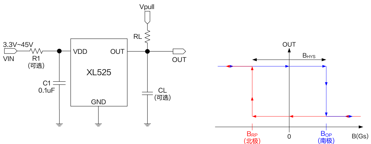
图 1. XL525 典型应用示意图和输出特性曲线
