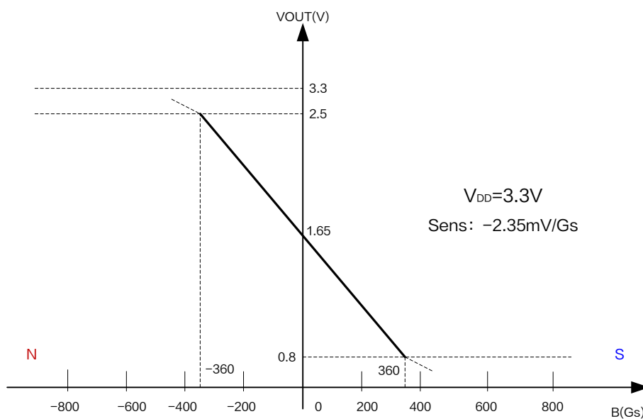
图 5.XL47Z 输出特性曲线 ( V_{DD} = 3.3\text{V} )
