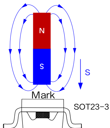
图 4.XL47Z 测试示意图
