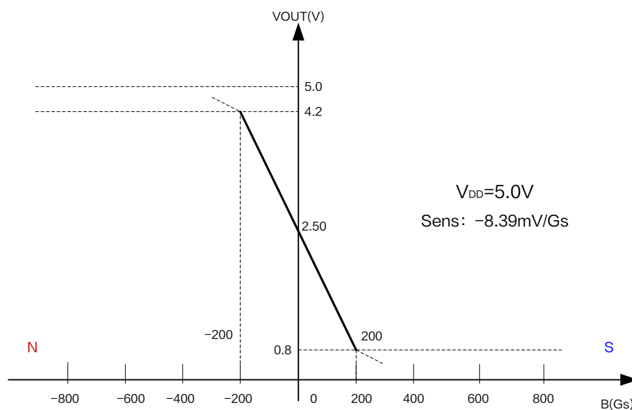
图 6.XL47Z 输出特性曲线 ( V_{DD} = 5.0V )
