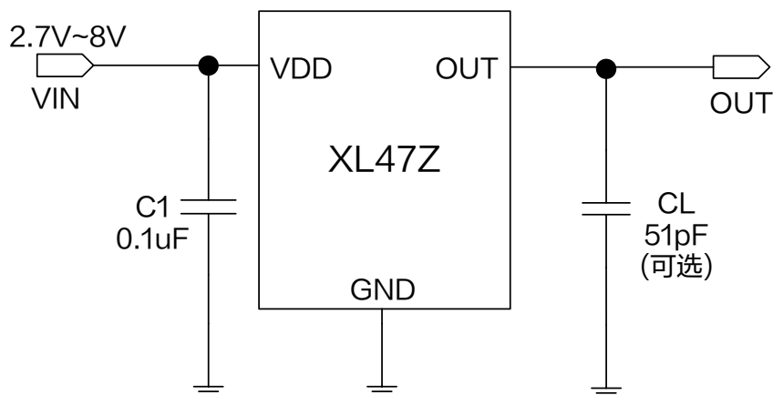
图 1.XL47Z 典型应用示意图
