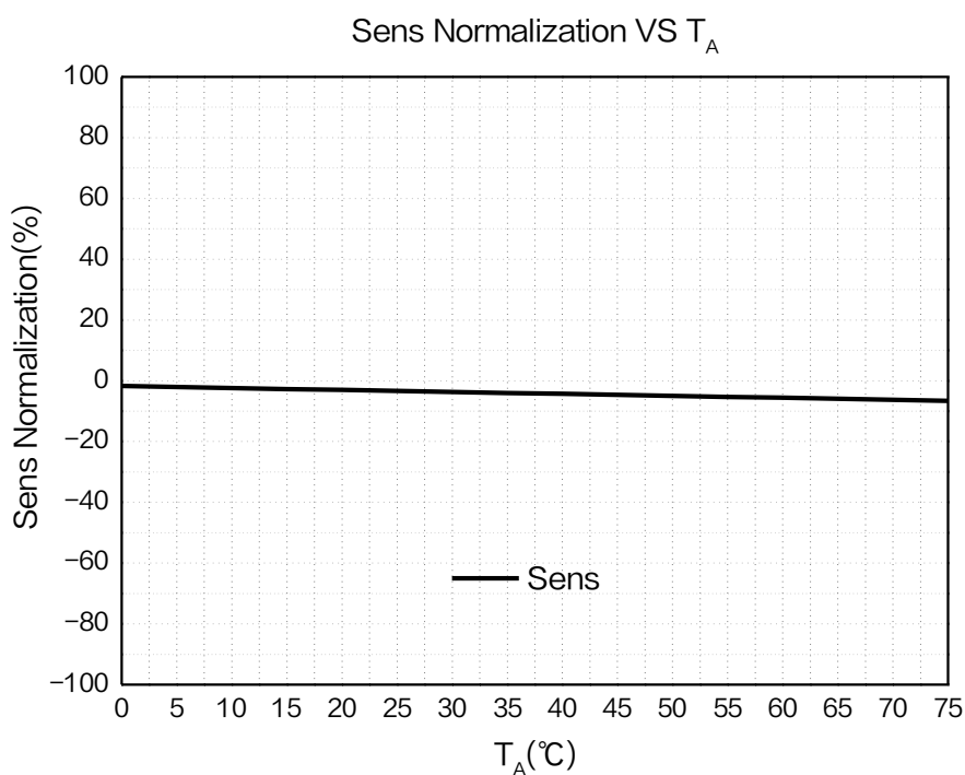
图 7.XL47Z 灵敏度随温度变化曲线 ( V_{DD} = 3.3V )
