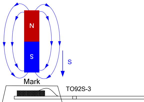
图 4. XL47T 测试示意图
