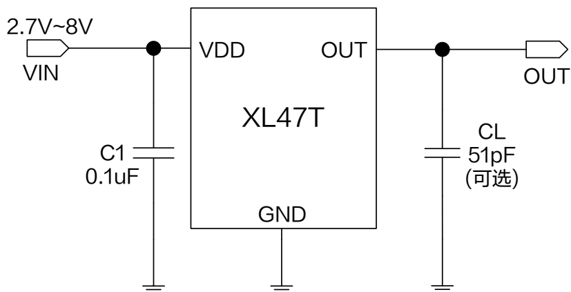
图 1. XL47T 典型应用示意图
