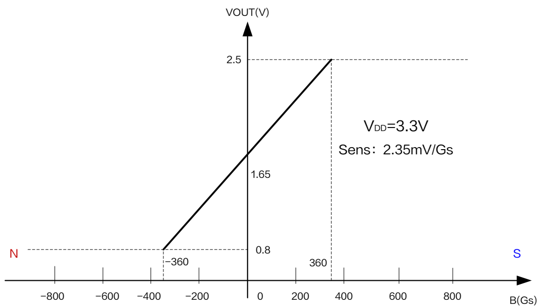
图 5. XL47T 输出特性曲线
