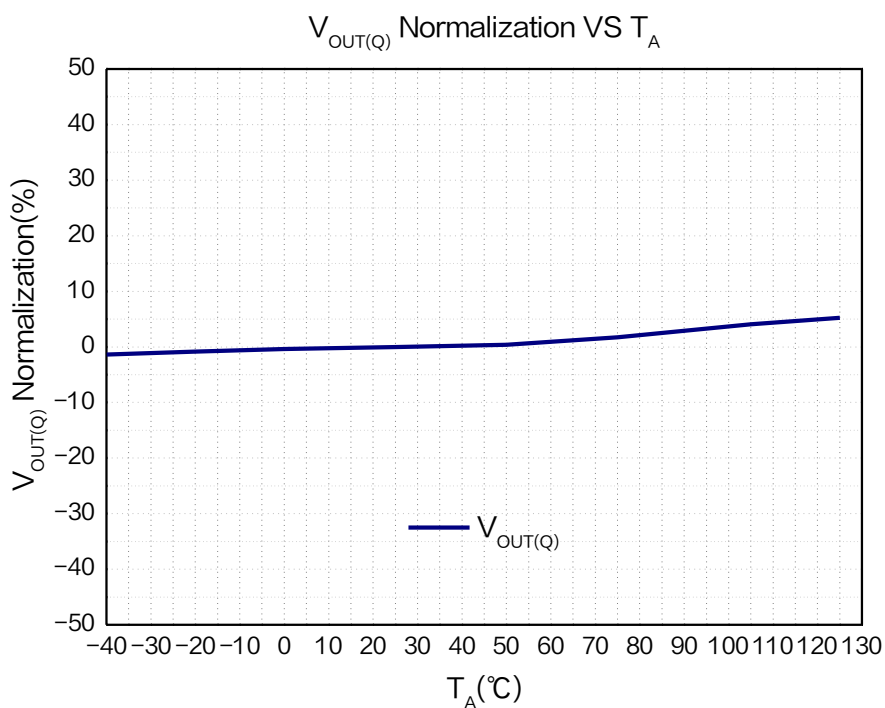
图 9.XL47E 静态输出电压随温度变化曲线 ( V_{DD} = 5.0V )
