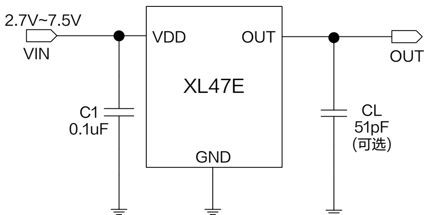
图 1.XL47E 典型应用示意图
