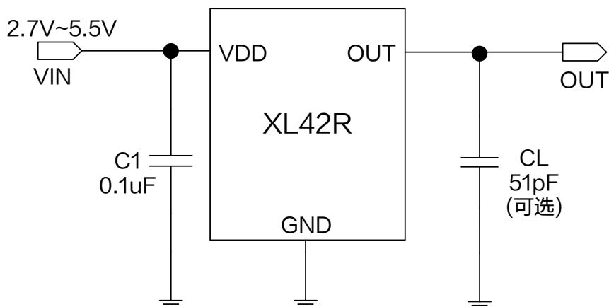
图 1.XL42R 典型应用示意图
