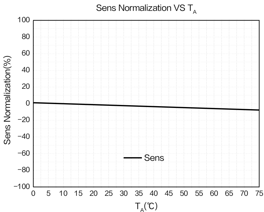
图 7.XL42R 灵敏度随温度变化曲线 ( V_{DD} = 3.3V )
