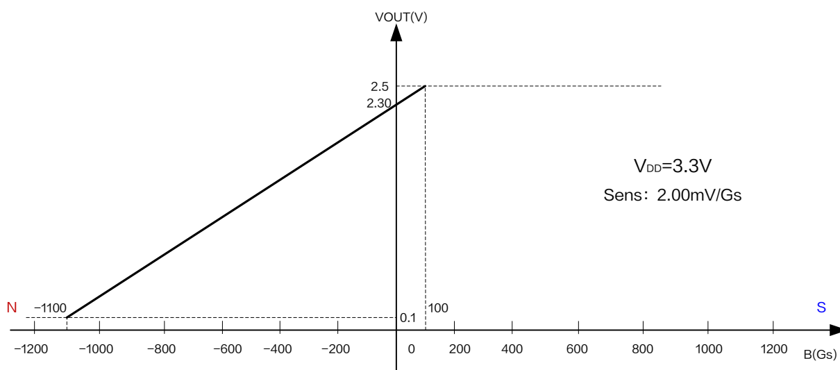
图 5.XL42R 输出特性曲线 ( V_{DD} = 3.3\text{V} )
