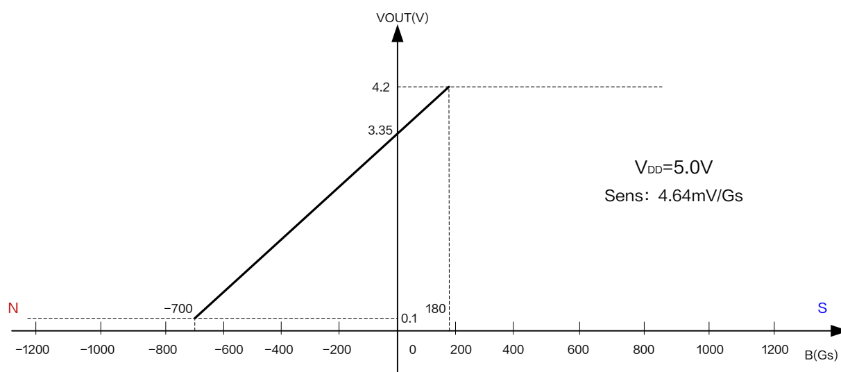
图 6.XL42R 输出特性曲线 ( V_{DD} = 5.0V )
