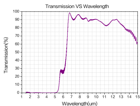
图5. 波长透射率
