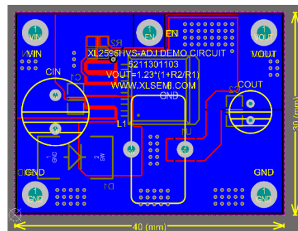
ADJ版本PCB底层截图
