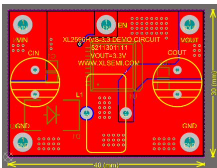
固定版本PCB顶层截图 (以3.3V版本为例)
