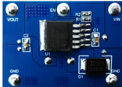
ADJ版本实物图反面
