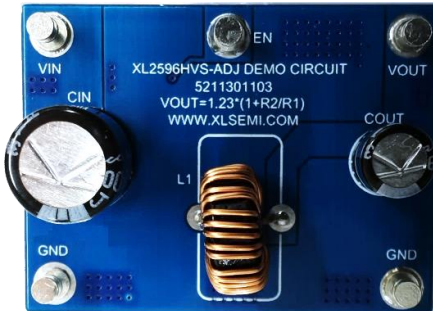
ADJ版本实物图正面
