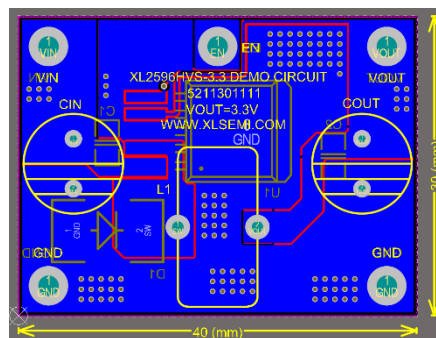
固定版本PCB底层截图 (以3.3V版本为例)
