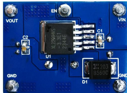
固定版本实物图反面 (以3.3V版本为例)
