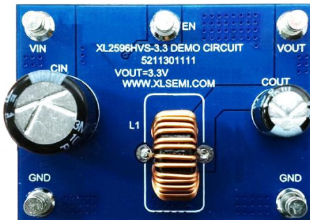
固定版本实物图正面 (以3.3V版本为例)
