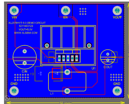
固定版本PCB底层截图 (以5.0V版本为例)
