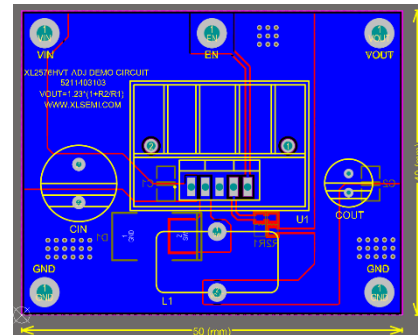
ADJ版本PCB底层截图
