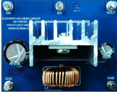
ADJ版本实物图正面
