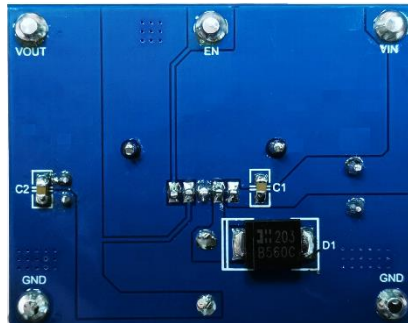
固定版本实物图反面 (以5.0V版本为例)
