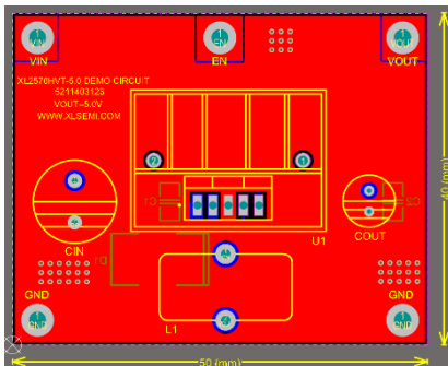
固定版本PCB顶层截图 (以5.0V版本为例)
