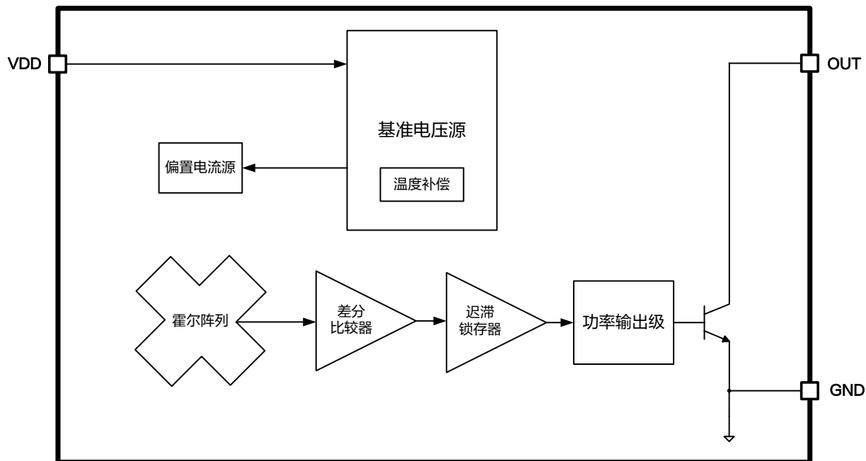
图 3. XL557 功能方框图
