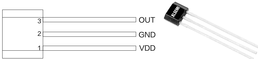
图 2. XL557 引脚配置
