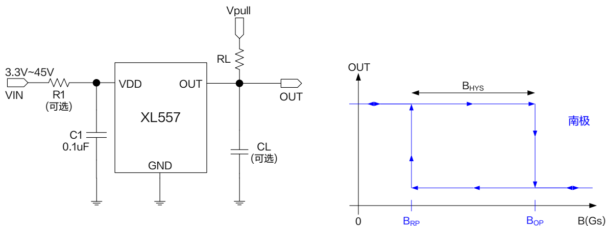
图 1. XL557 典型应用示意图和输出特性曲线
