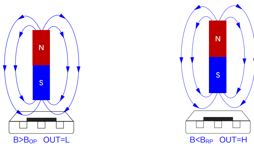
图 4. XL557 磁场方向定义图
