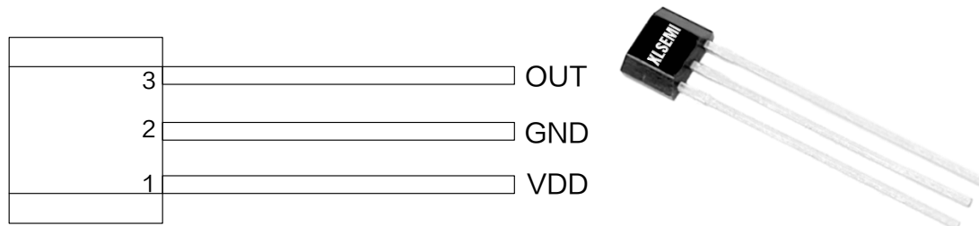
图 2. XL555 引脚配置
