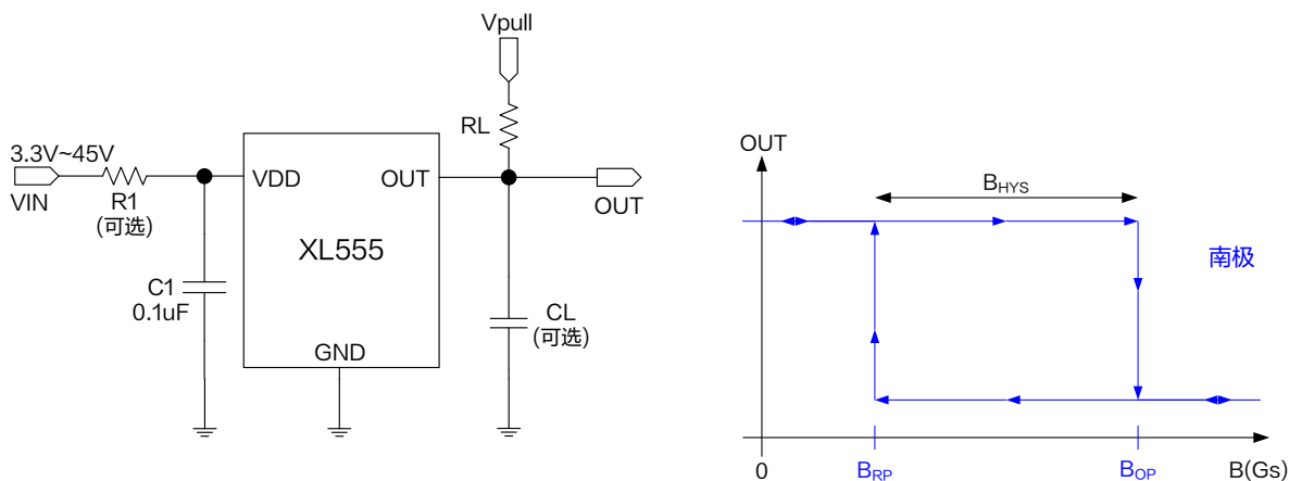
图 1. XL555 典型应用示意图和输出特性曲线
