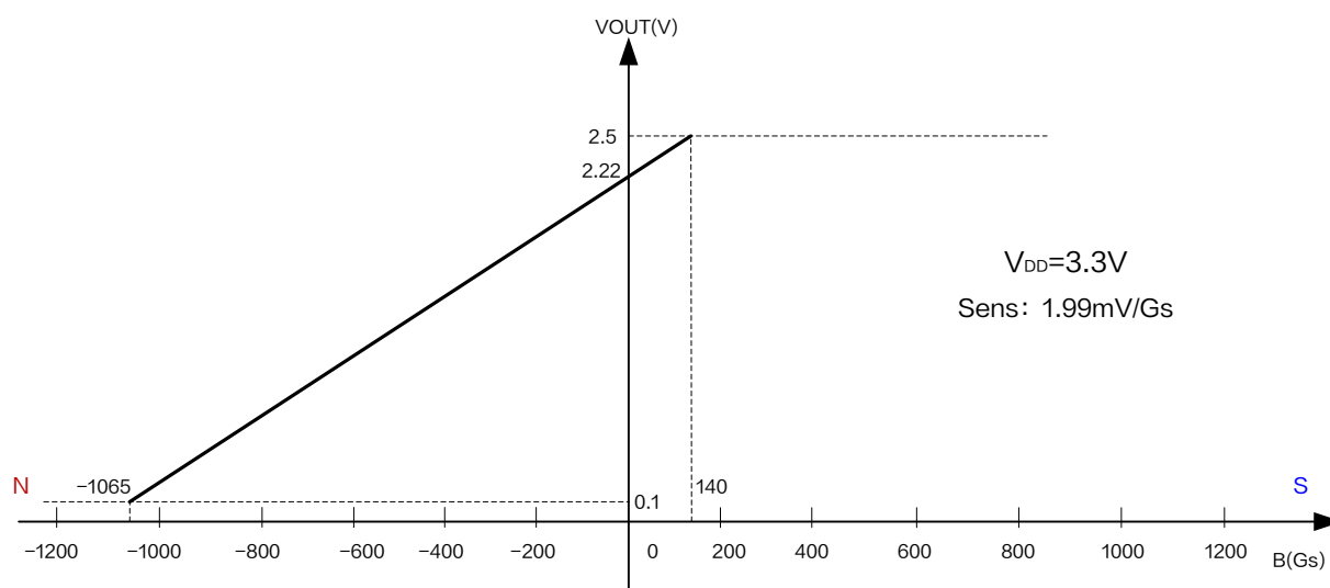
图 5.XL47 输出特性曲线 ( V_{DD} = 3.3\text{V} )
