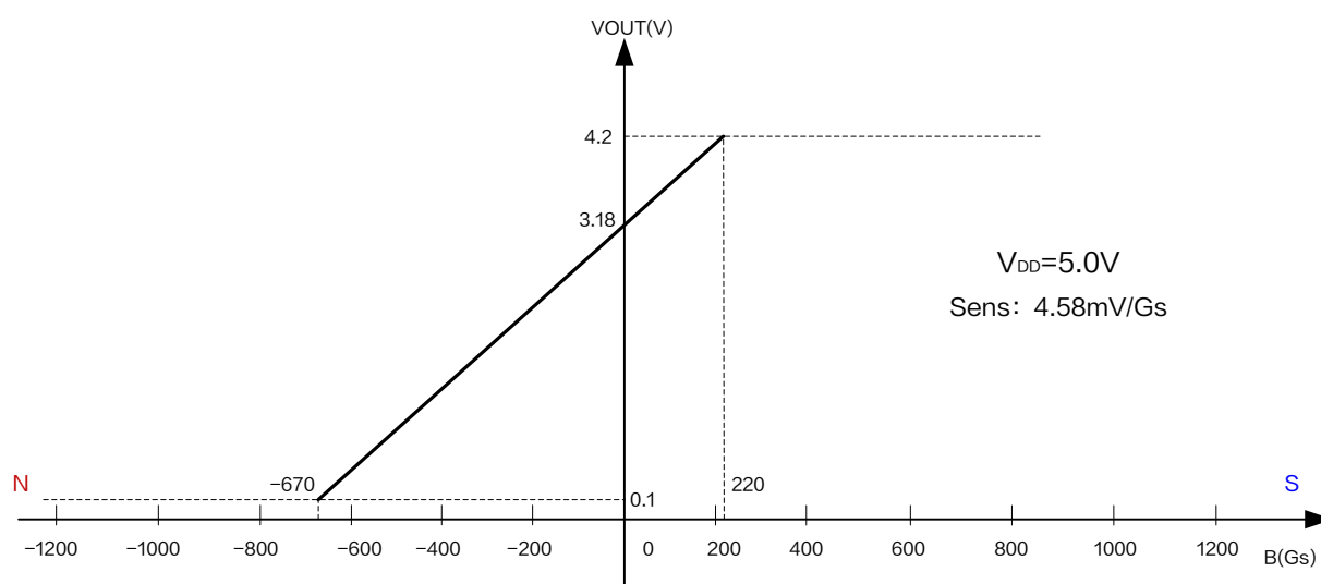
图 6.XL47 输出特性曲线 ( V_{DD} = 5.0V )
