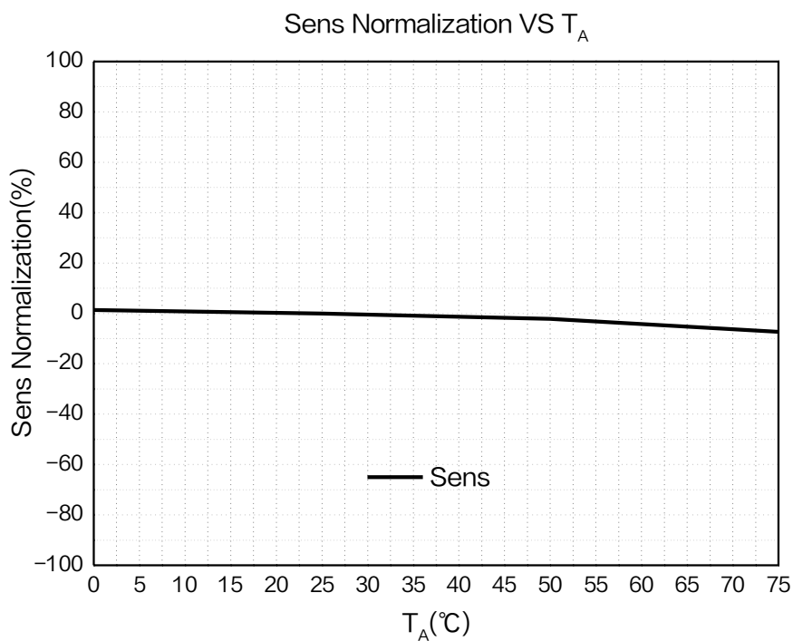
图 7.XL47 灵敏度随温度变化曲线 ( V_{DD} = 3.3V )
