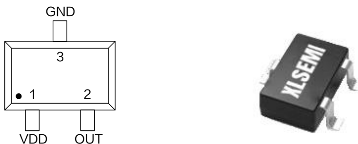
图 2.XL47 引脚配置
