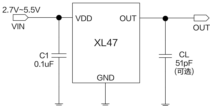
图 1.XL47 典型应用示意图
