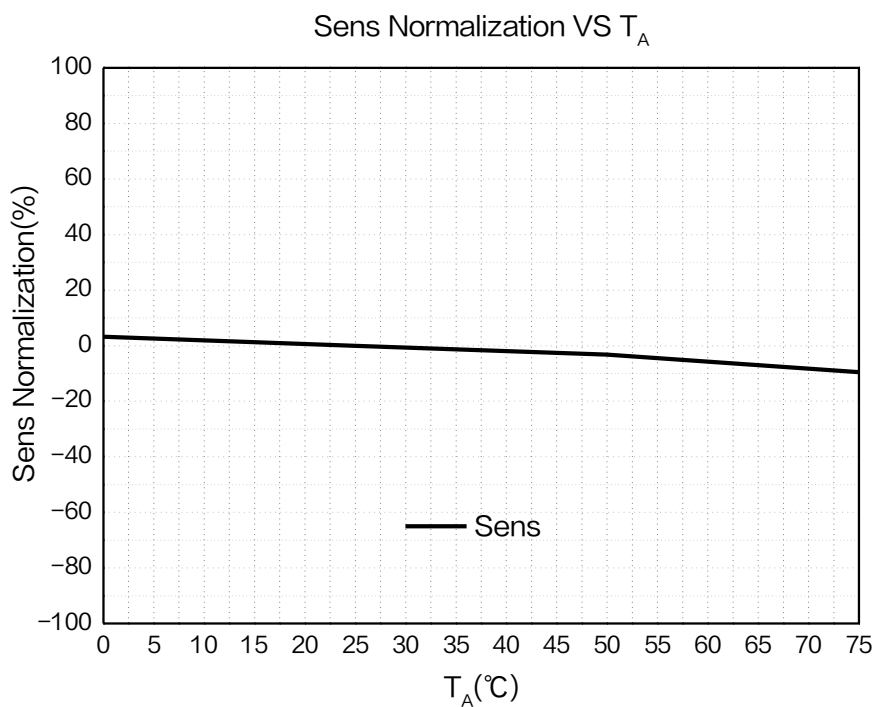
图 7.XL46 灵敏度随温度变化曲线 ( V_{DD} = 3.3V )
