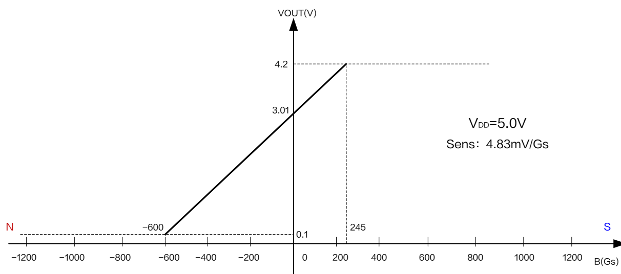
图 6.XL46 输出特性曲线 ( V_{DD} = 5.0V )
