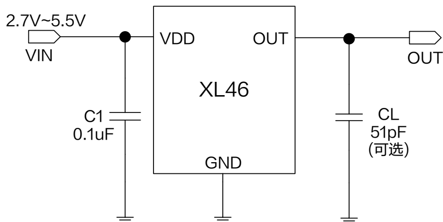
图 1.XL46 典型应用示意图
