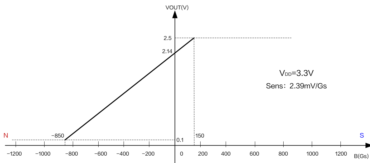
图 5.XL46 输出特性曲线 ( V_{DD} = 3.3V )
