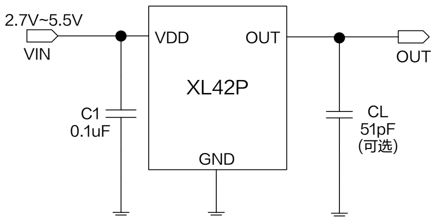
图 1.XL42P 典型应用示意图
