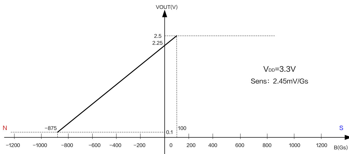
图 5.XL42P 输出特性曲线 ( V_{DD} = 3.3\text{V} )
