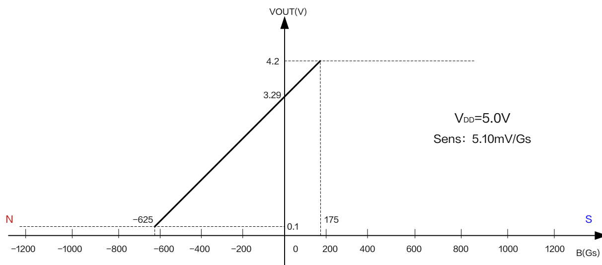
图 6.XL42P 输出特性曲线 ( V_{DD} = 5.0V )
