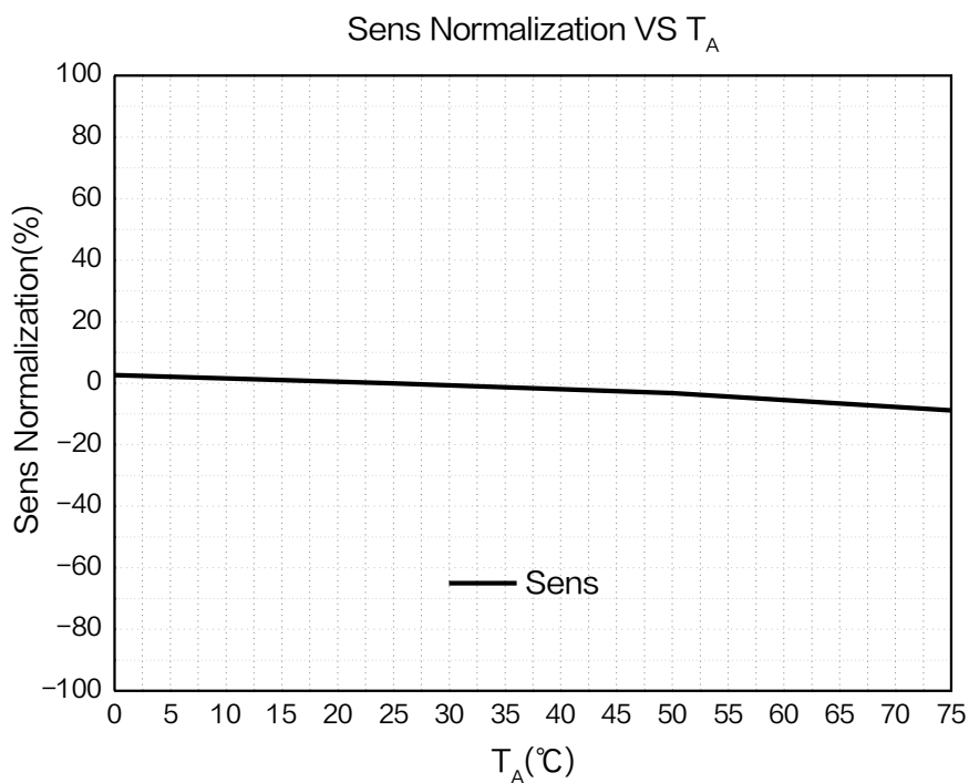
图 7.XL42P 灵敏度随温度变化曲线 ( V_{DD} = 3.3V )
